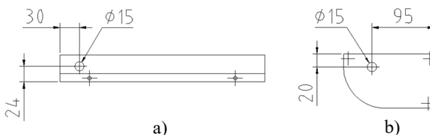
Figur 1. Placering av hål i montageplatta.
