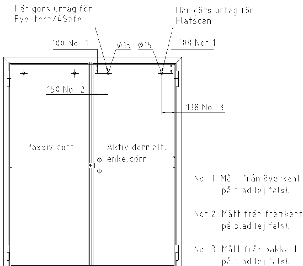
Figur 2. Urtag i dörrblad.
