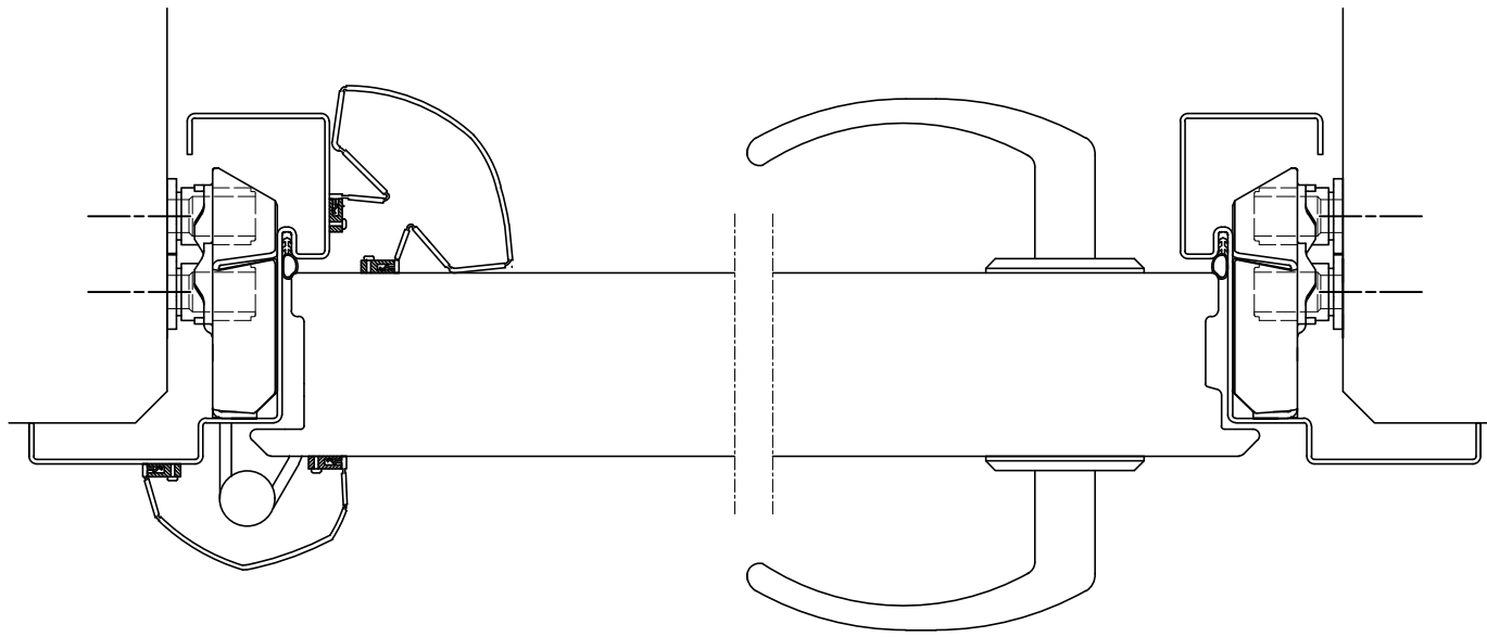
Utanpåliggande klämskydd
