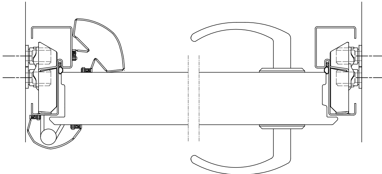
Utanpåliggande klämskydd
